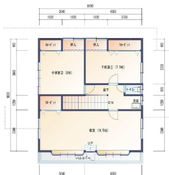
2階 平面図
